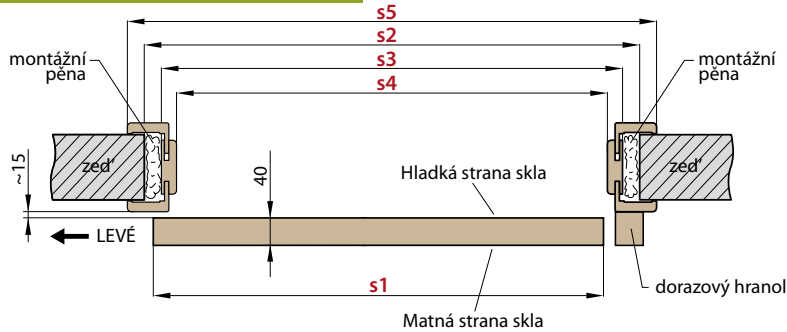
PD1S (levé dveře)
