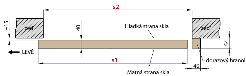
PD2S (levé a pravé dveře)
