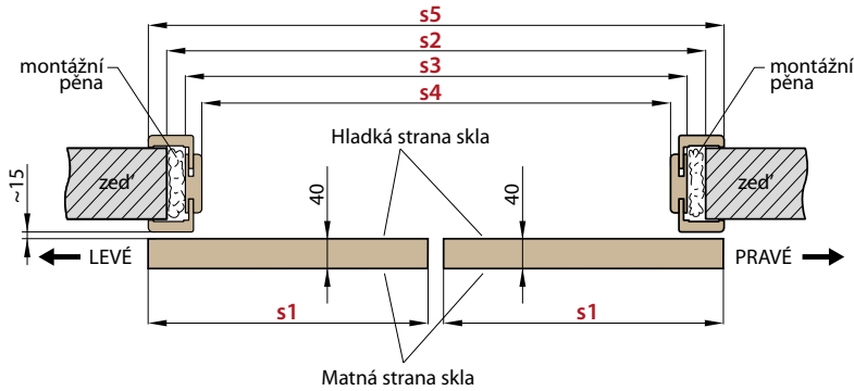
PD2S (levé a pravé dveře)
