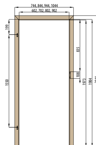
OBLOŽKOVÁ ZÁRUBĚŇ PRO CELOSKLENĚNÉ DVEŘE
