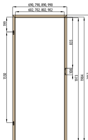
RÁMOVÁ ZÁRUBĚŇ PRO CELOSKLENĚNÉ DVEŘE
