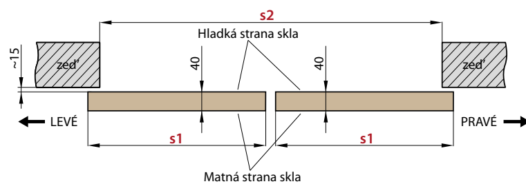
PD2S (levé a pravé dveře)
