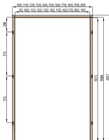
RÁMOVÁ ZÁRUBĚŇ PRO DVOUKŘÍDLÉ DVEŘE
