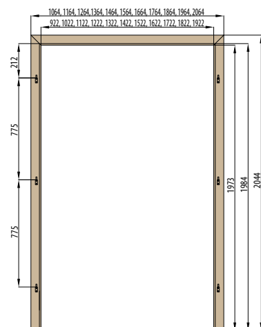
OBLOŽKOVÁ ZÁRUBĚŇ PRO DVOUKŘÍDLÉ DVEŘE
