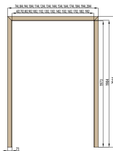
OBLOŽKOVÁ ZÁRUBĚŇ TYPU TUNEL (SLEPÁ)
