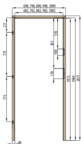
RÁMOVÁ ZÁRUBĚŇ
